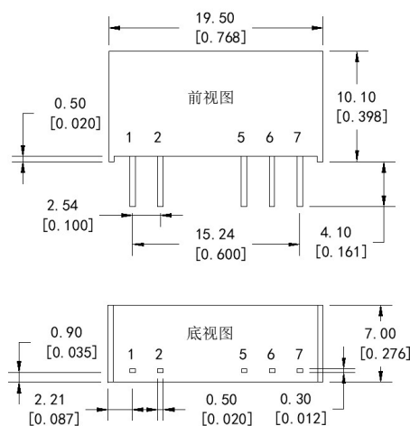
封装尺寸图
